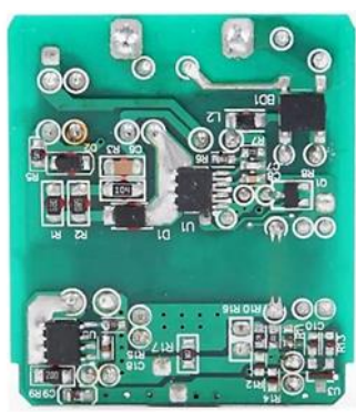
内置MOS 18W PD快充方案
